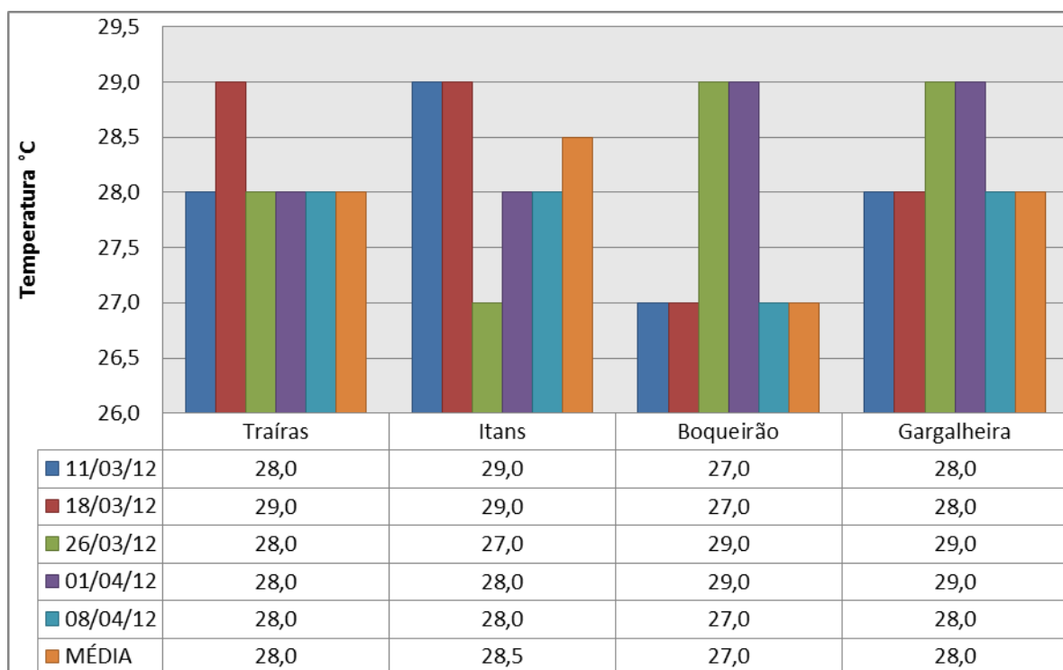
Figura 14. Resultados da temperatura das águas dos reservatórios da Região Seridó.
