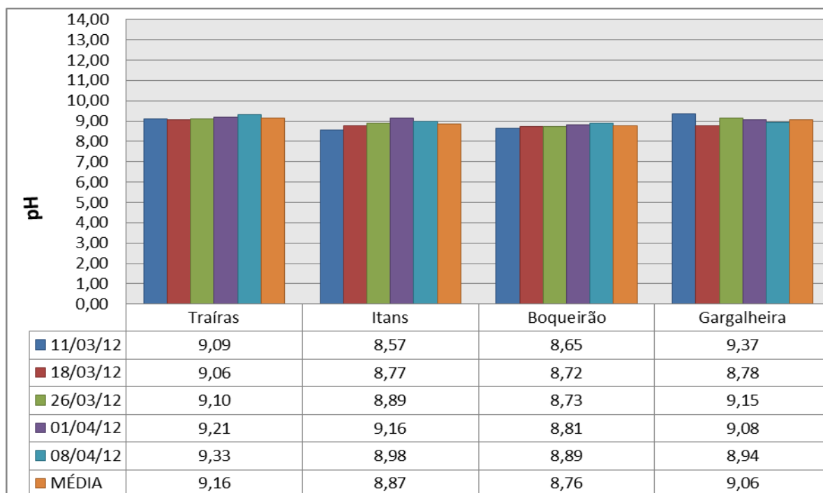
Figura 16. Resultados do pH das águas dos reservatórios da Região Seridó.
