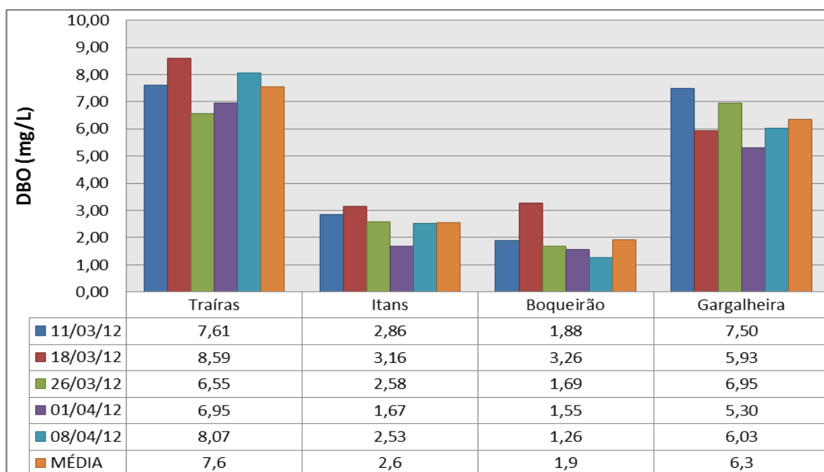
Figura 20. Resultados da DBO das águas dos reservatórios da Região Seridó.
