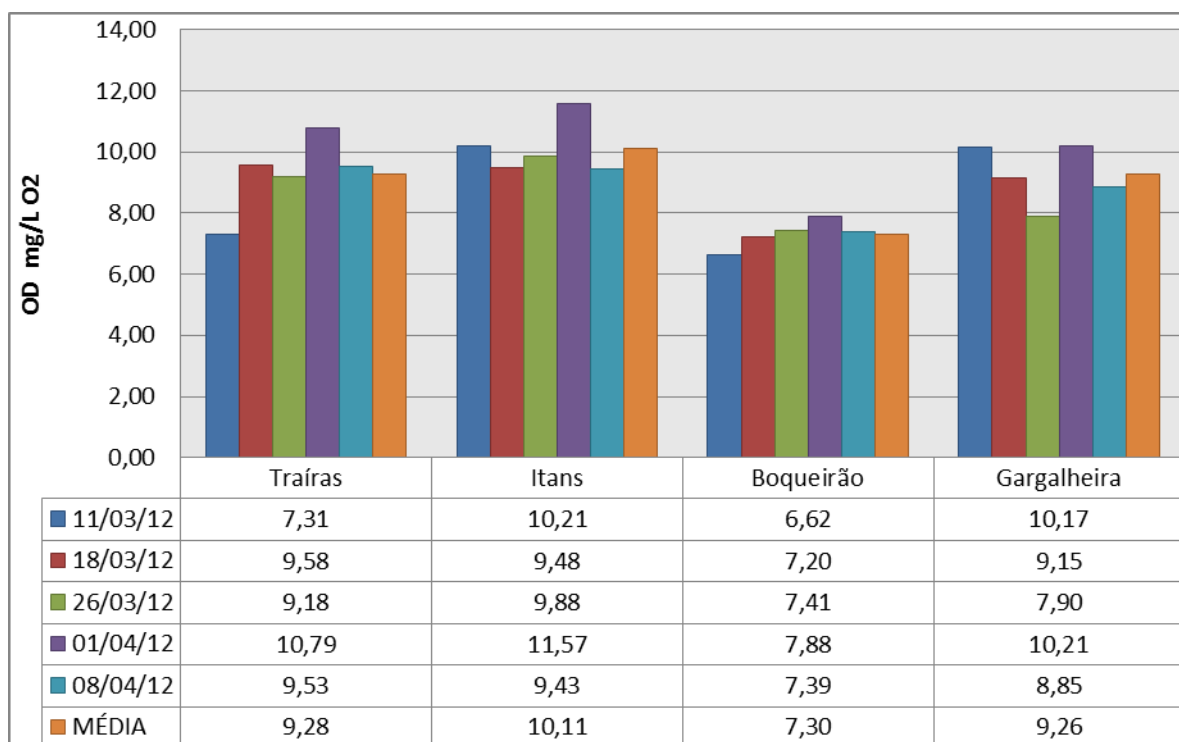
Figura 18. Resultados de oxigênio dissolvido das águas dos reservatórios da Região Seridó.
