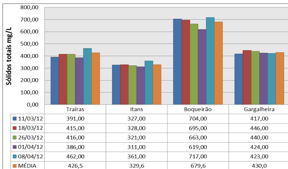
Figura 32. Resultados de sólidos totais na água dos reservatórios da Região Seridó.
