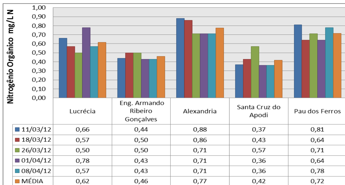
Figura 29. Resultados de Nitrogênio Orgânico das águas dos reservatórios da Região Oeste.
