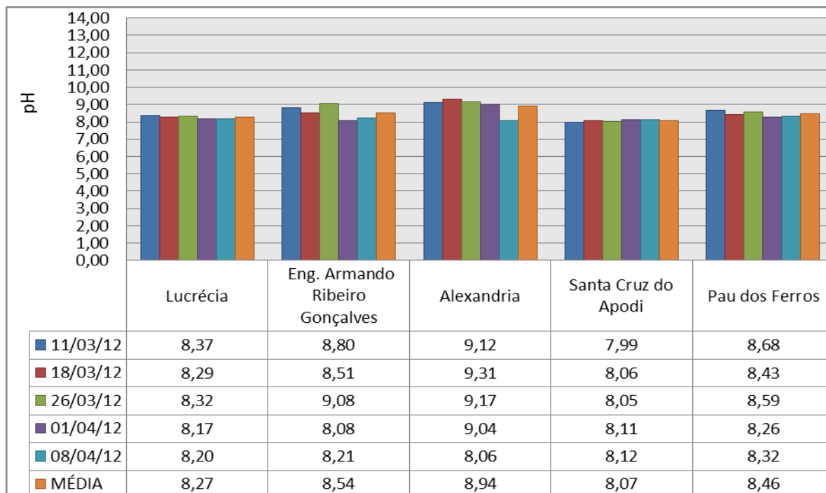
Figura 15. Resultados do pH das águas dos reservatórios da Região Oeste.
