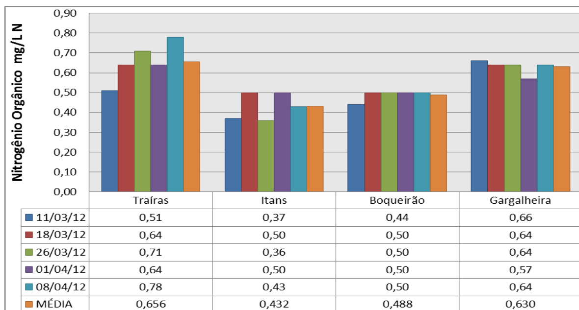
Figura 30. Resultados de Nitrogênio Orgânico das águas dos reservatórios da Região Seridó.
