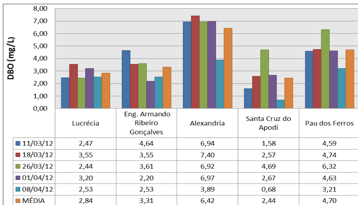
Figura 19. Resultados da DBO das águas dos reservatórios da Região Oeste.
