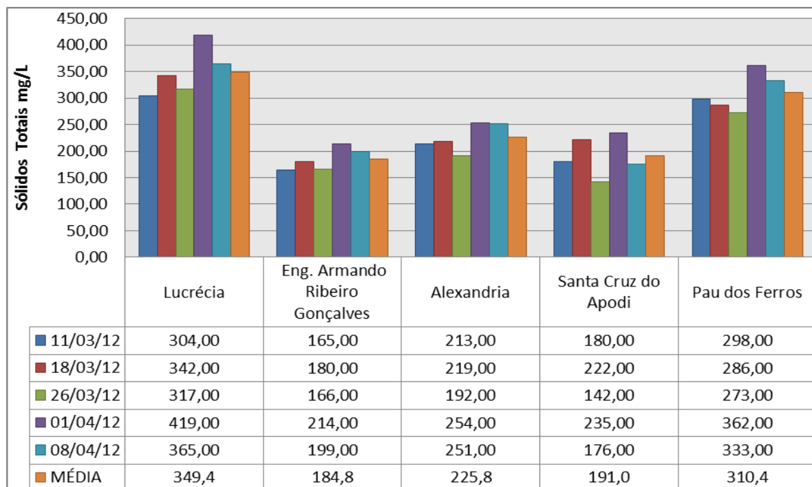
Figura 31. Resultados de sólidos totais das águas dos reservatórios da Região Oeste.
